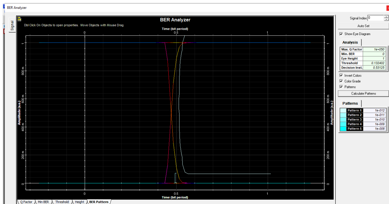
3.8 Сурет - Бос кеңістіктегі оптикалық байланыстың көз диаграммасы
