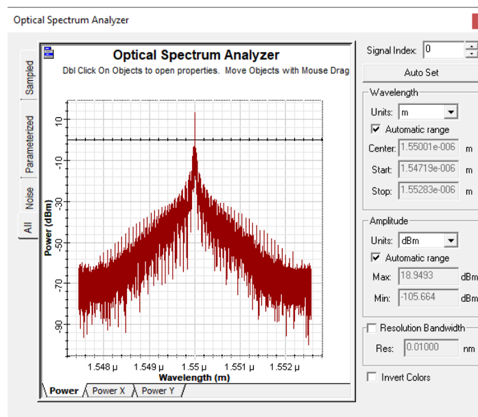
3.7 Сурет - Оптикалық спекторының толқын ұзындығы мен қуатқа тәуелді графигі
