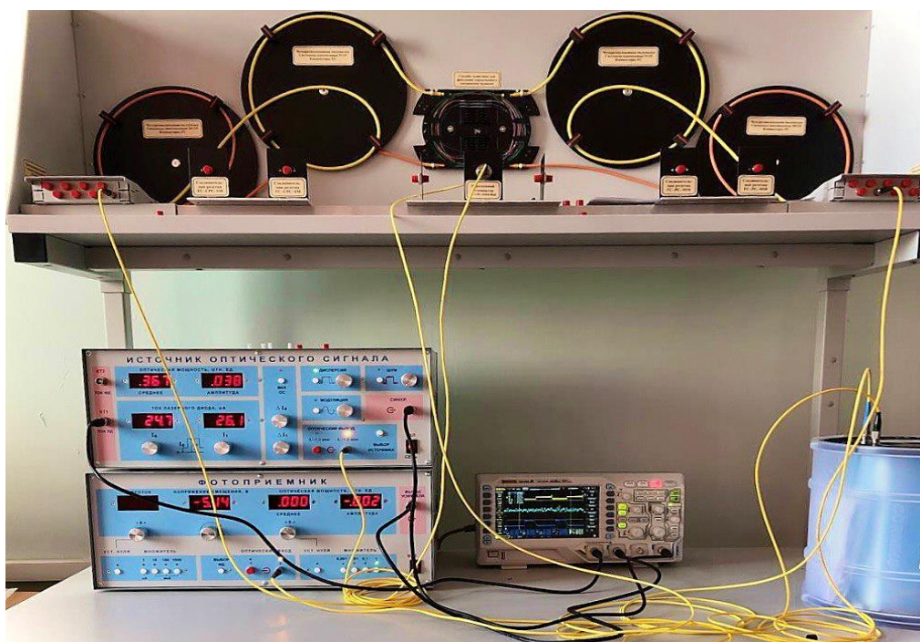
2.4 Сурет - Оптикалық сызықтық жол моделінің блогы
