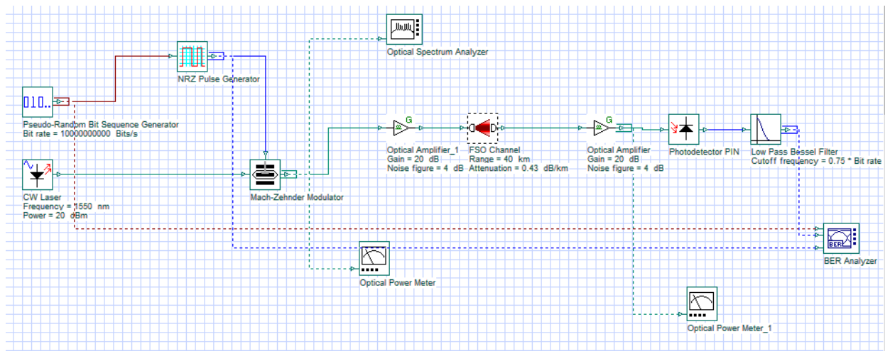
3.5 Сурет - Optisystem программалық жүйесінде бос кеңістіктегі оптикалық байланыс көмегімен дерек алмасу моделі [40]
