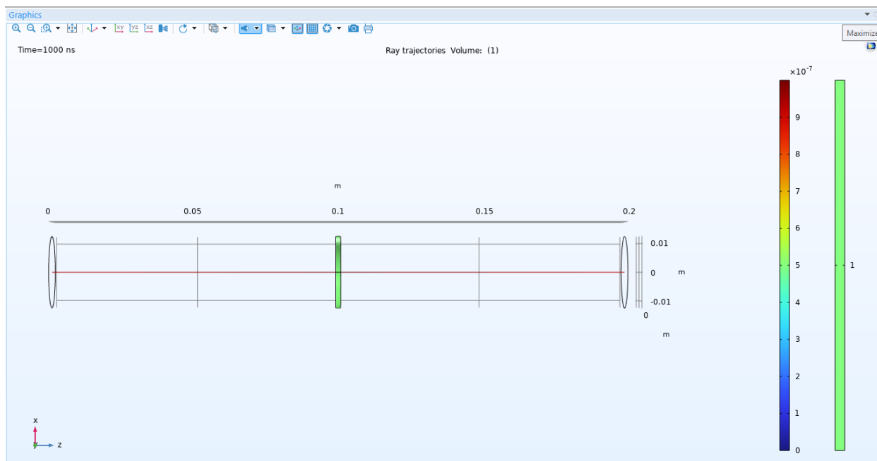
3.1 Сурет - COMSOL Multiphysics бағдарламалық жүйесінде 3Д сәулелік оптика моделінің тік көрінісі
